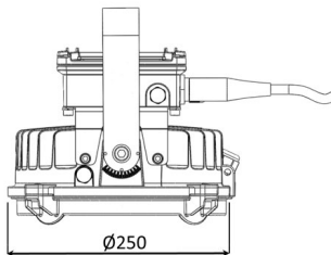
A 275 B 239 (mm)
